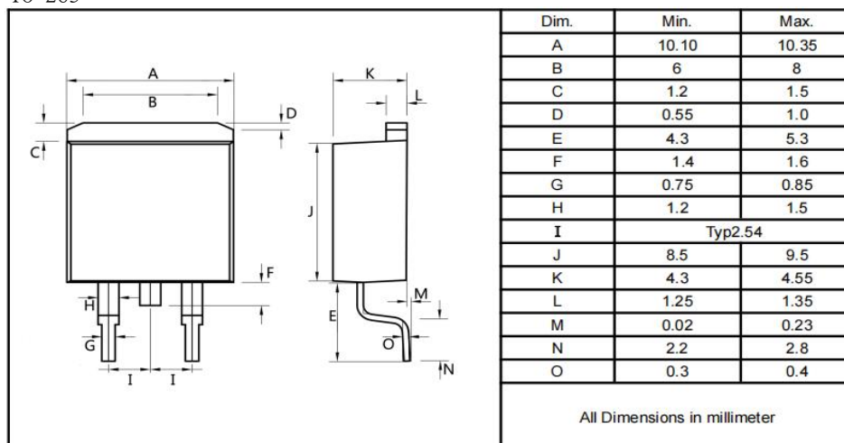
TO-263
